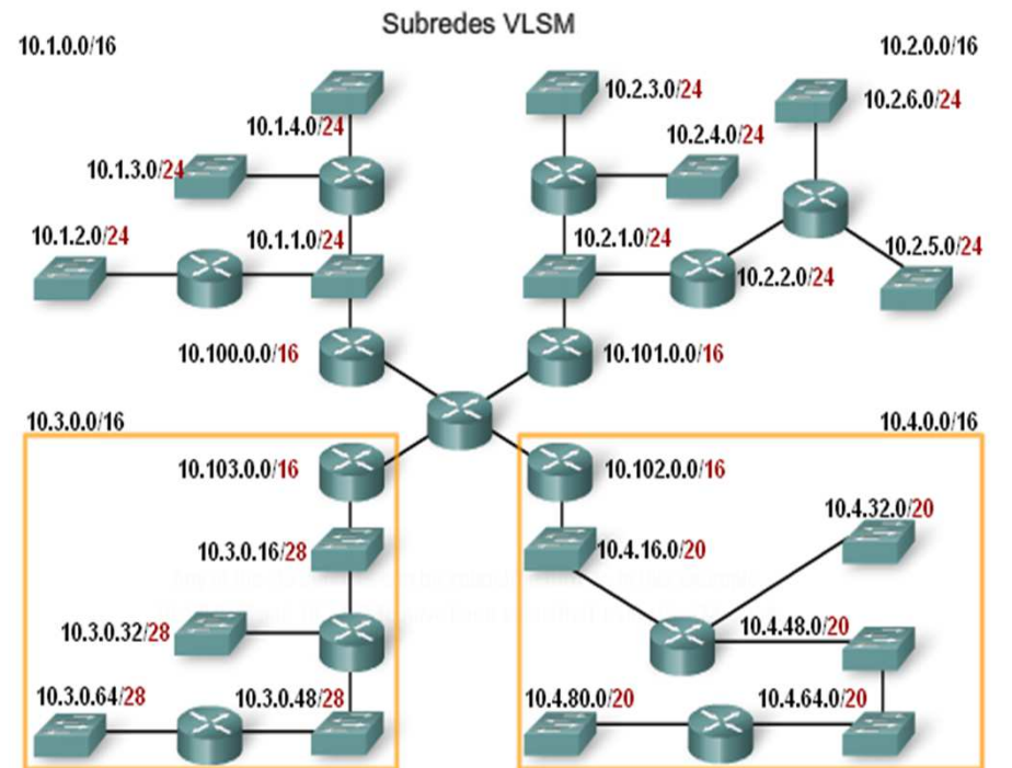
En este ejemplo, 10.3.0.0/16 ha sido dividida en subredes utilizando la máscara /28 y 10.4.0.0/16 ha sido dividida en subredes utilizando la máscara /20.
